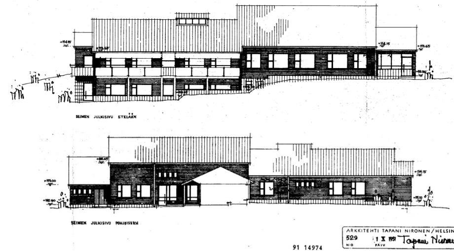
Kalevan lastentalon seimiosan julkisivut etelään ja pohjoiseen. Arkkitehti Tapani Nirosen alkuperäisissä lupakuvissa vuodelta 1951 on nähtävissä seimen etelälaapeella ikkunat, joita ei kuitenkaan toteutettu, kuten sivujen 4 ja 9 kuvista voi todeta.
